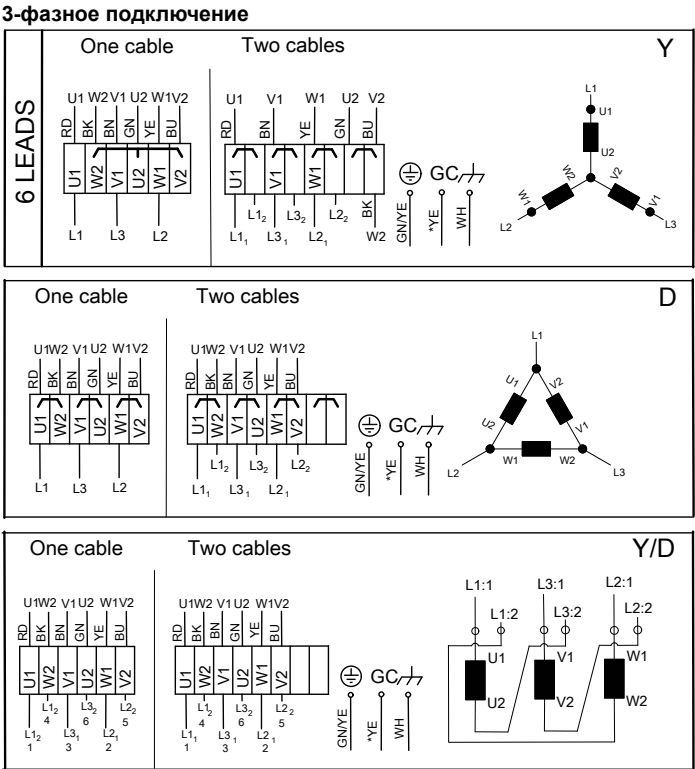
Рис. 6: 6 проводов
