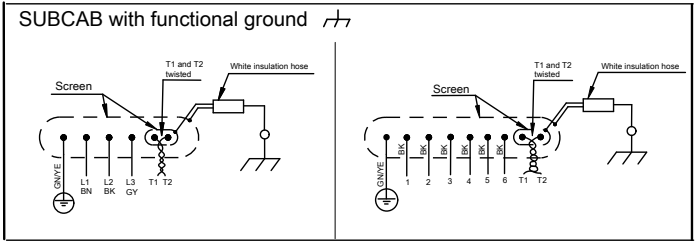
Рис. 7: Функциональное заземление
