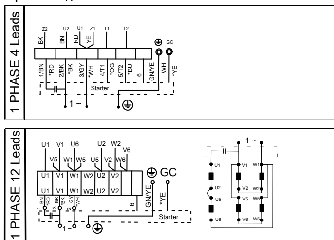
Рис. 10: 4 провода, 12 проводов
