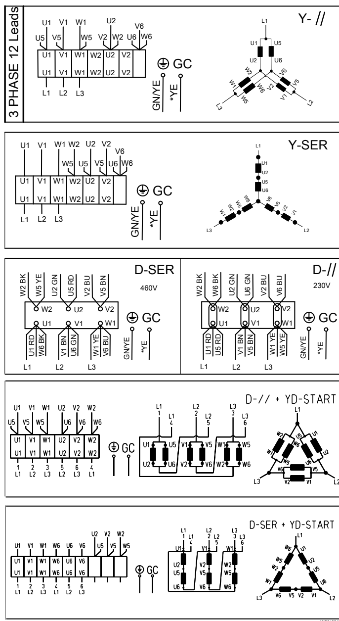
Рис. 9: 12 проводов
