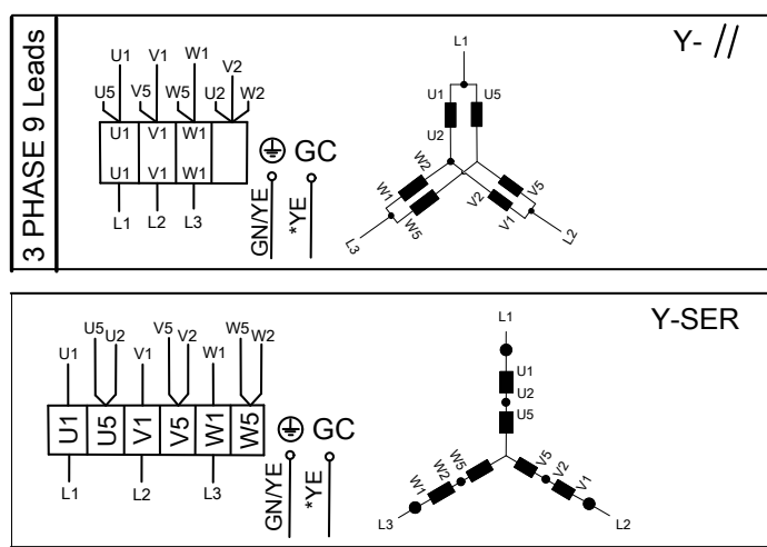
Рис. 8: 9 проводов
