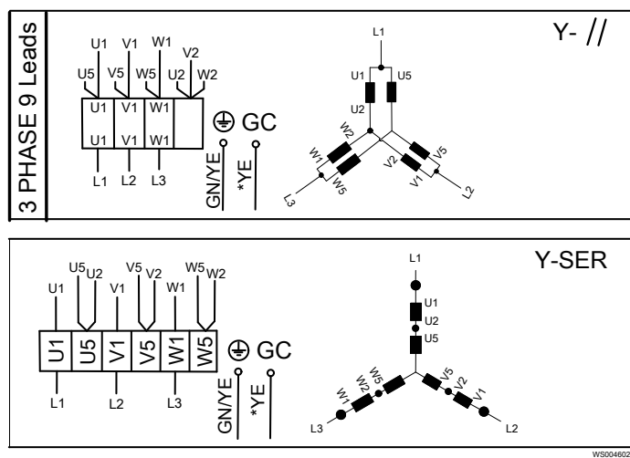
Рис. 8: 9 проводов
