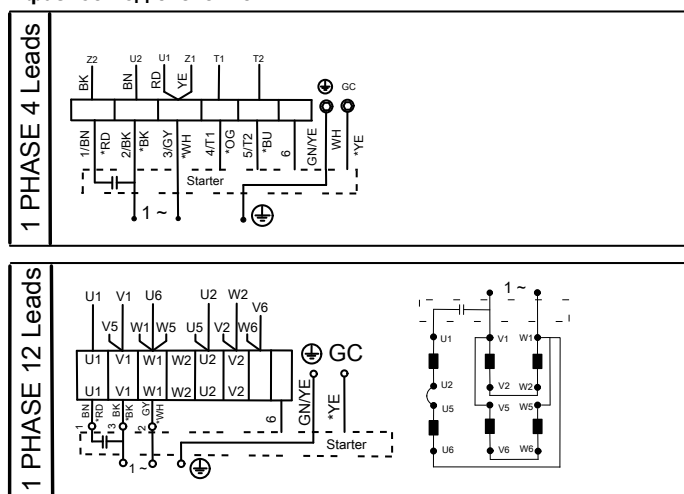
Рис. 10: 4 провода, 12 проводов
