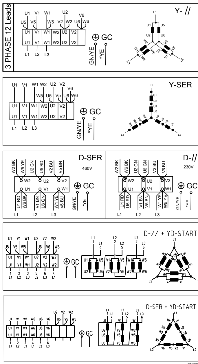
Рис. 9: 12 проводов
