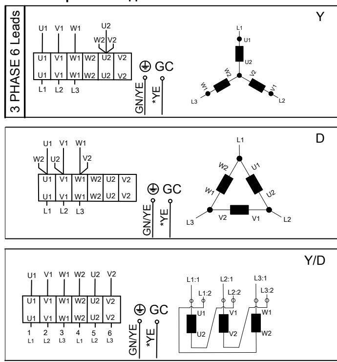
Рис. 7: 6 проводов
