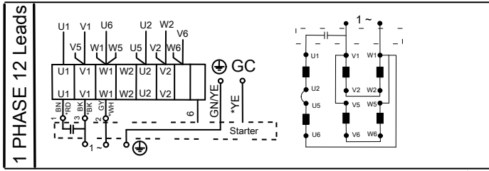
Рис. 10: 4 провода, 12 проводов
