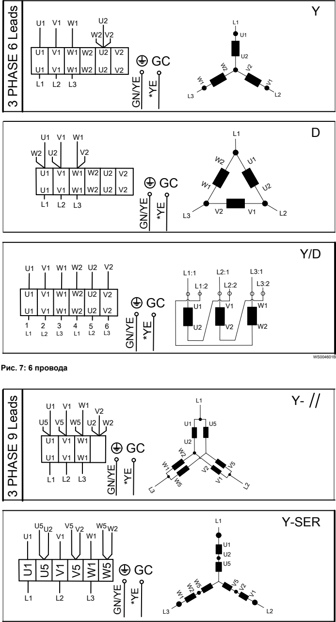
Рис. 8: 9 проводов
