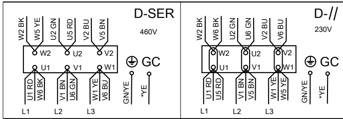
Рис. 9: 12 проводов
