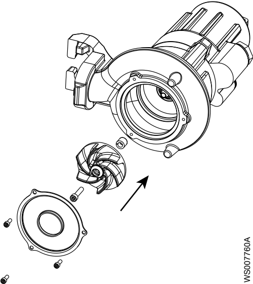
Рис. 12: Вихревой насос
